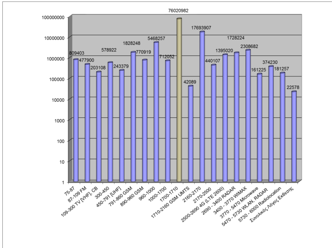
Εικόνα 6. Πόσες φορές κάτω από το θεσμοθετημένο όριο είναι η ηλεκτρομαγνητική επιβάρυνση
