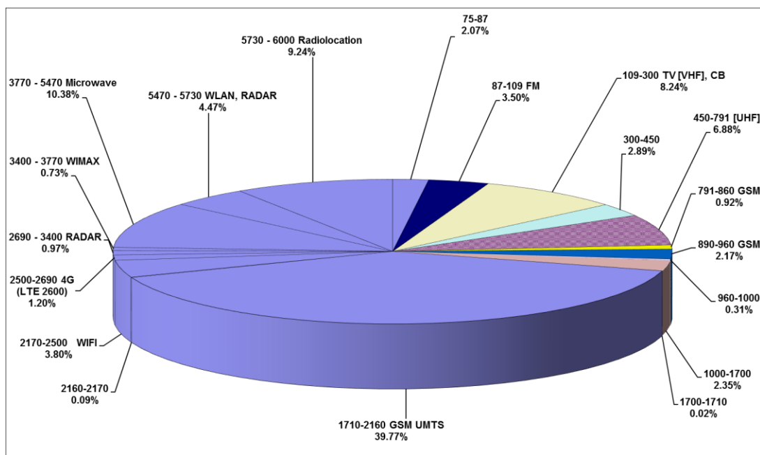
Εικόνα 7. Συνεισφορά κάθε υποπεριοχής φάσματος στη συνολική ηλεκτρομαγνητική επιβάρυνση
